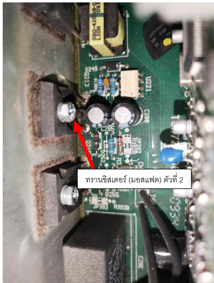
อุปกรณ์ทรานซิสเตอร์ (มอสเฟต) ตัวที่ 2 ระเบิด
