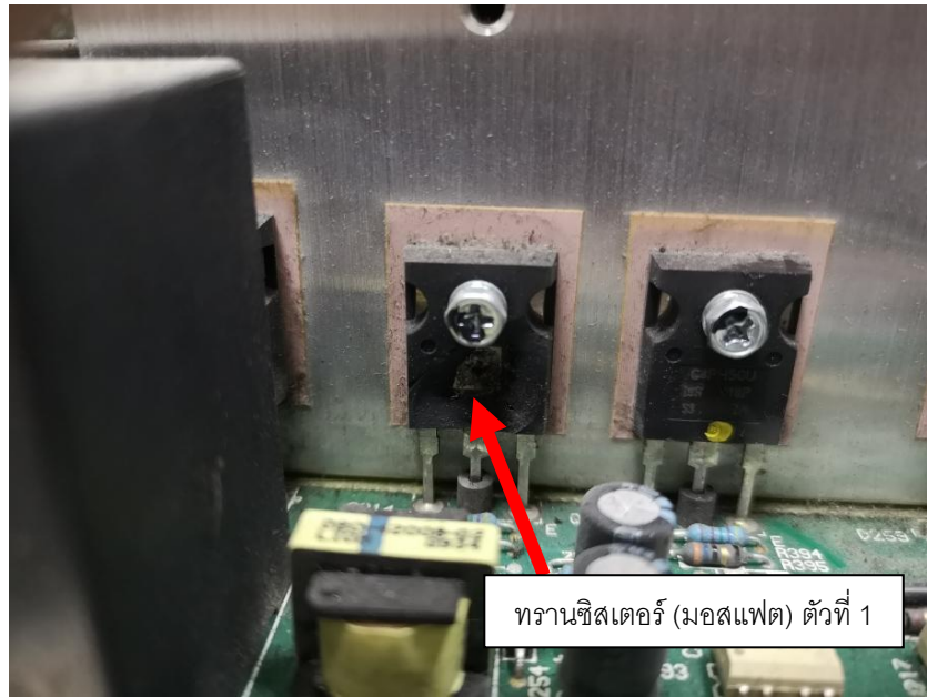
อุปกรณ์ทรานซิสเตอร์ (มอสเฟต) ตัวที่ 1 ระเบิด
